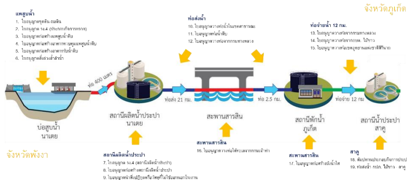
รูปภาพแนวการต่อเชื่อมท่อของ GS กับแนวท่อของ กปภ.
