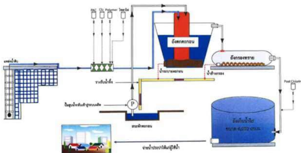
รูปภาพขั้นตอนการผลิตน้ำประปาของ GS
