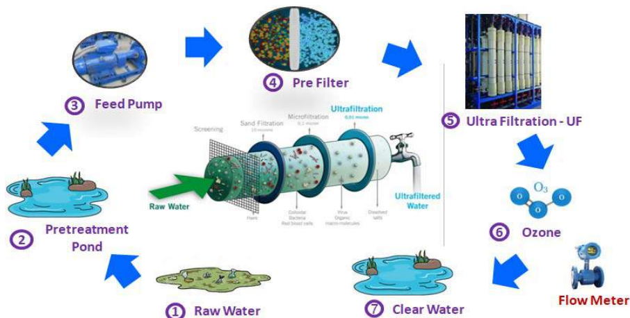
กระบวนการบำบัดน้ำด้วยระบบอัลตราฟิเตรชัน (Ultrafiltration) และกำจัดเชื้อด้วยระบบโอโซน (Ozone)
